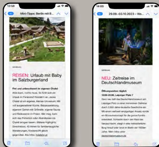
Beispiel: Mobile-Ansicht
